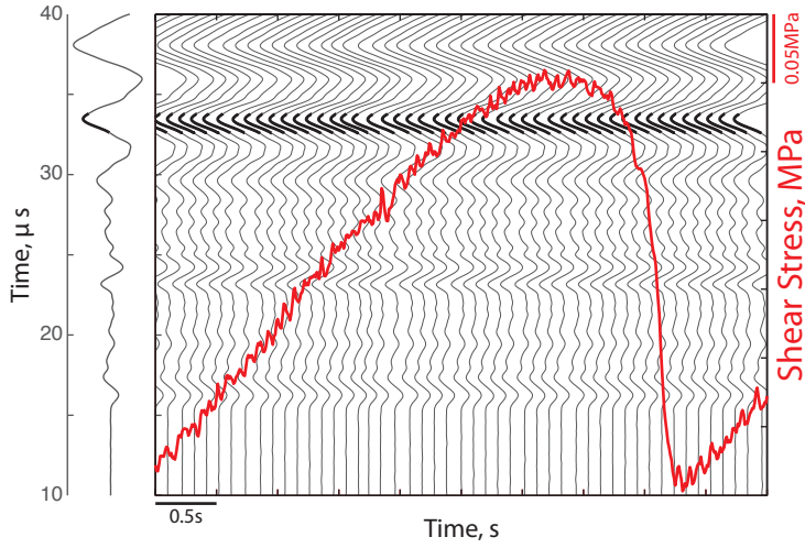
Onde sismiche analizzate durante il ciclo sismico
